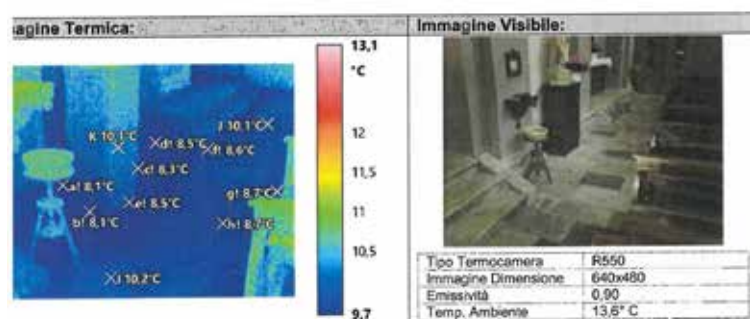
Significativa immagine termica a destra dell'altare di s. Antonio: la parte evidenziata in blu riconosce la presenza di umidità nella zona.
